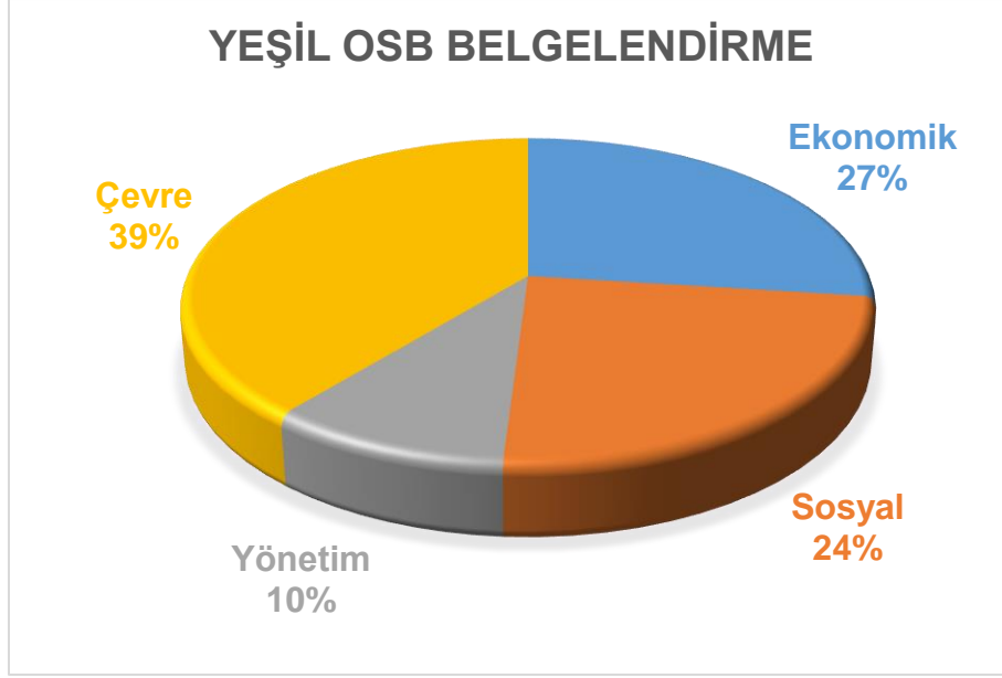
Şekil 1. Puanlandırma Dağılımı
